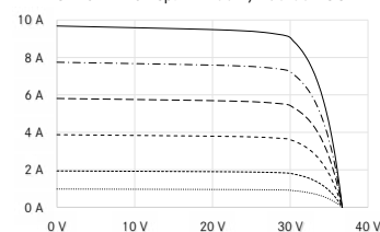
UI-Kennlinie Bsp. LX-280M/156-60+ GG
