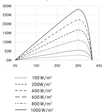
UP-Kennlinie Bsp. LX-280M/156-60+ GG
