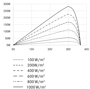
UP-Kennlinie Bsp. LX-280M/156-60+ GG
