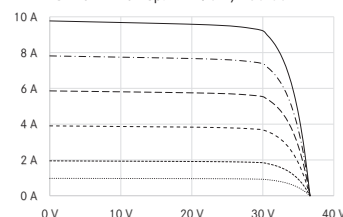
UI-Kennlinie Bsp. LX-290M/156-60+
